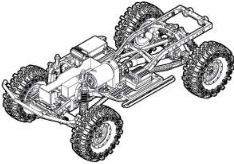
GS02 샤시 chassis
